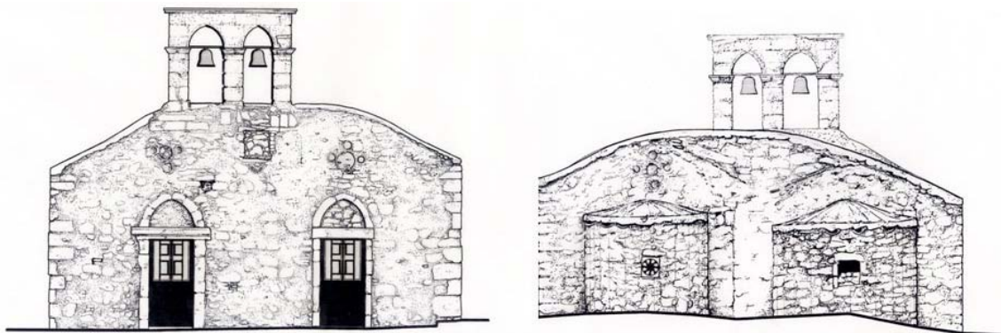
Εικ. 3. Σχεδιαστική αποτύπωση της ανατολικής και της δυτικής όψης του Καθολικού της Μονής Χαλέπας.
